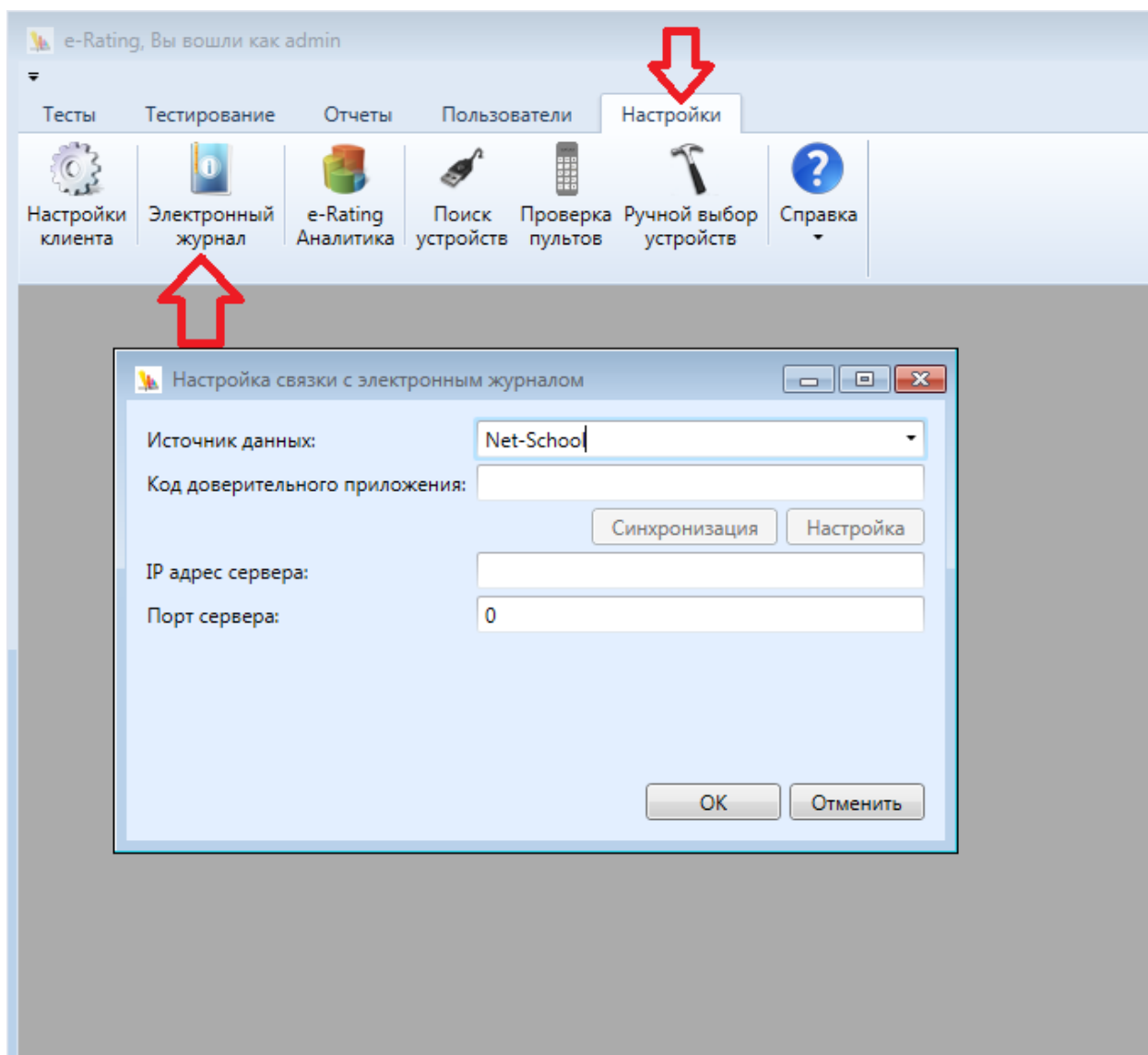
Рис. 1 – окно настроек
