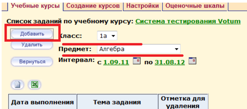
Рис. 5 – Добавление задания
