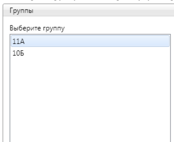
Рис. 2 – Выбор группы
